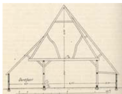
Binderkonstruktion der Scheune von 1755
