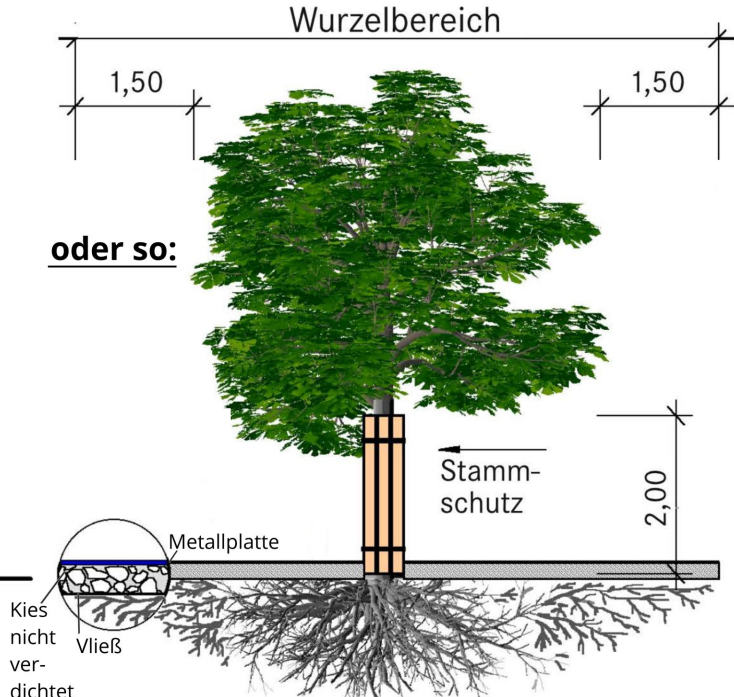
Wurzelschutz durch Lastverteilung (nur im abgestimmten Einzelfall und dann zeitlich begrenzt)
