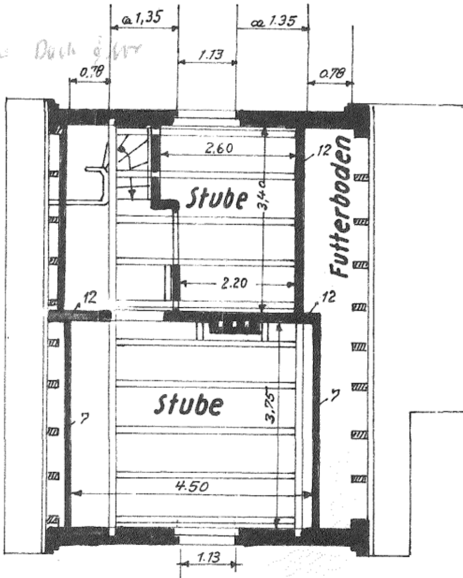
Dachgeschoß
